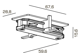
Стык внутренний
