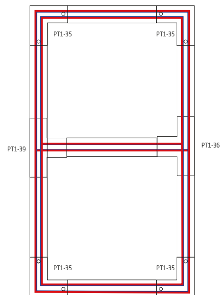
3. Прямоугольное соединение
