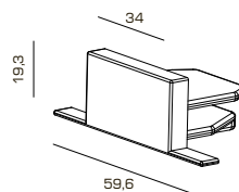
Заглушка
