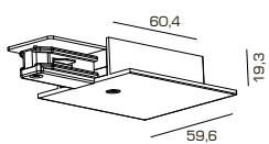
Токоподвод
